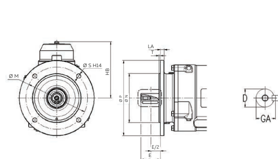
Mocowanie kołnierzone B5
