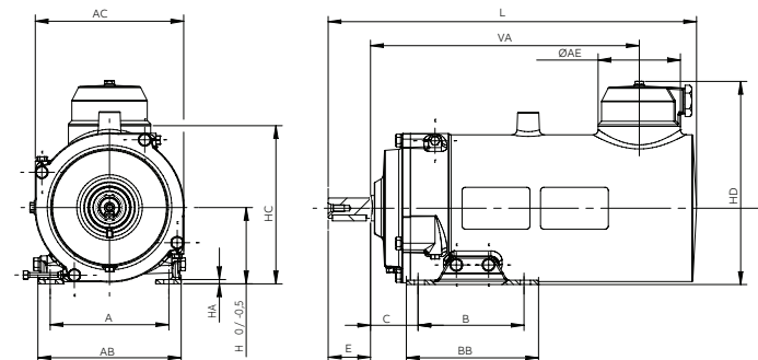
Mocowanie na łapach B3
